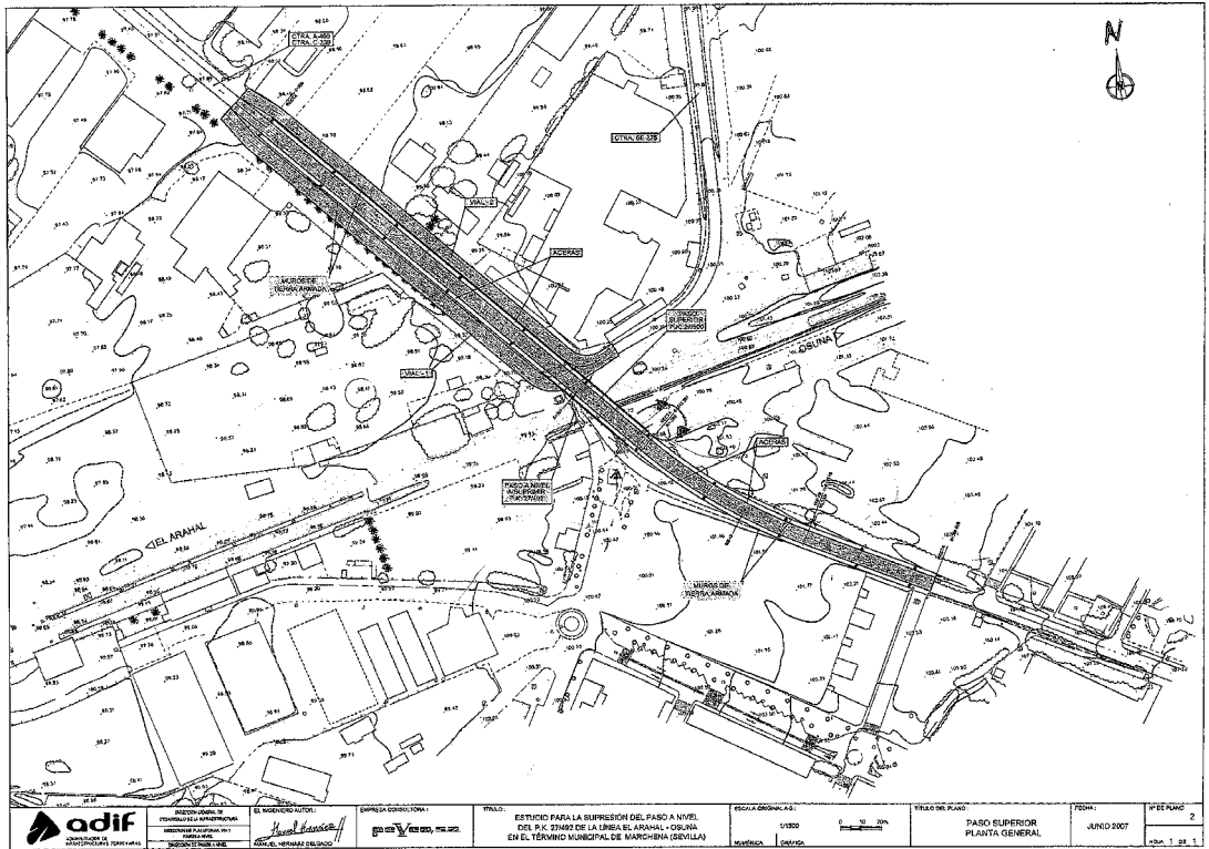
ESTUDIO PARA LA SUPRESIÓN DEL PASO A NIVEL FFCC ARAHAL-OSUNA CON CARRETERA DE CARMONA
